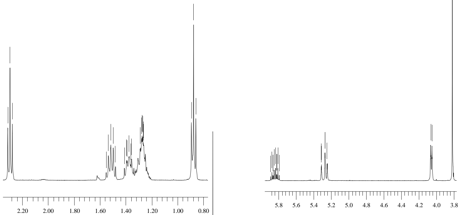
N -(Methoxycarbonyl)- N -(2-propenyl)-1,3-decadiynylamide #3122 step C
