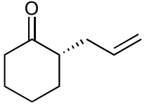
2-Allylcyclohexanone
