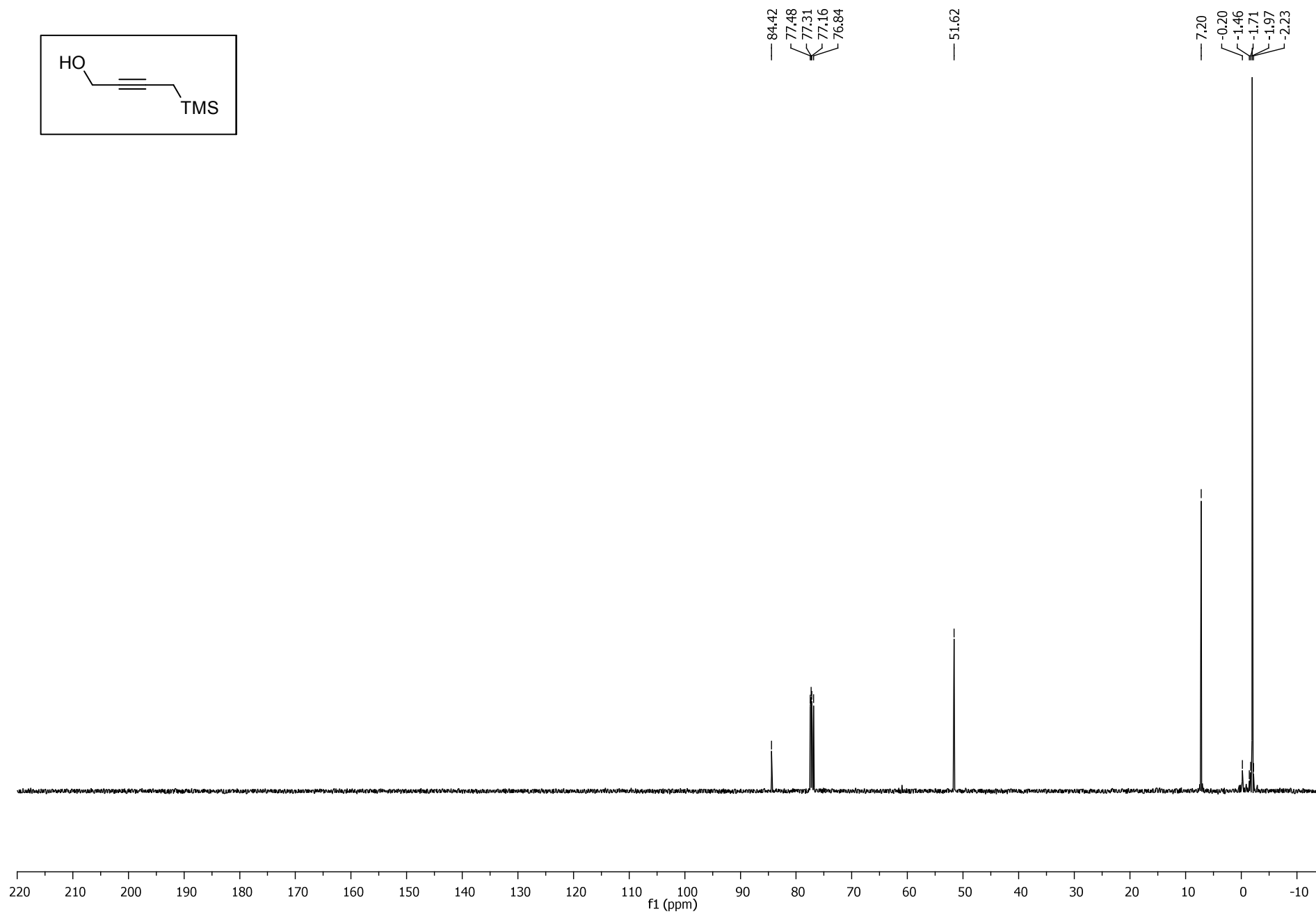
^{13}\text{C} NMR of 4-TRIMETHYLSILYL-2-BUTYN-1-OL
