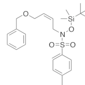
(Z)-N-(4-(benzyloxy)but-2-en-1-yl)- N-((tert-butyl dimethylsilyl)oxy)-4- methylbenzenesulfonamide
