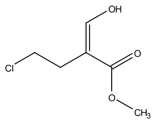
(Z)-1b
